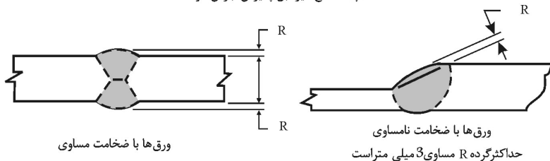
(ت) مقاطع قابل پذیرش جوش های شیاری
