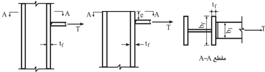
شکل ۱۰-۲-۹-۱۶ خمشی موضعی بال در مقابل نیروی متمرکز کششی
