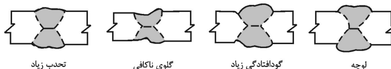
(ث) مقاطع غیر قابل پذیرش جوش گوشه
