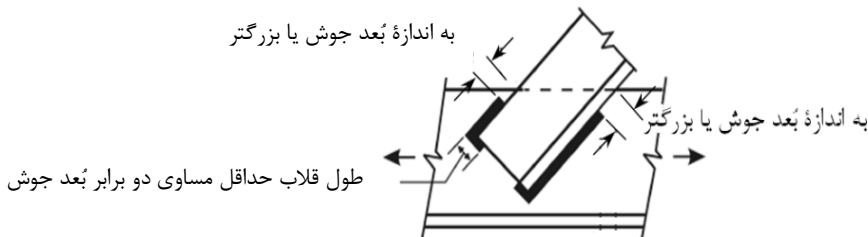
شکل ۹-۲-۱۰-۶ جوش گوشه در انتهای اعضای محوری
