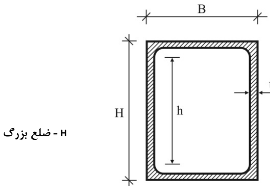
شکل ۱۰-۲-۷-۱ مقطع قوطی شکل
