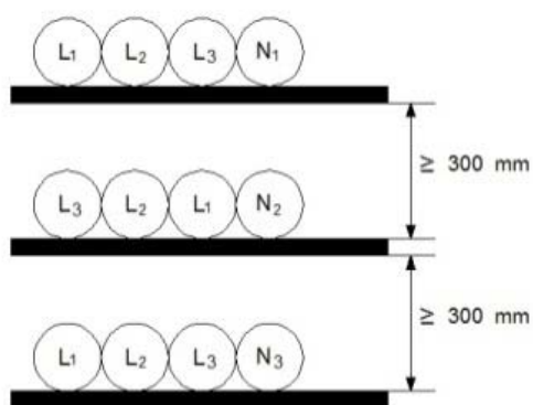
شکل ۷-۱۳-۱-۷-۱: آرایش چسبیده به هم در سه تراز و هر تراز به فاصله ۳۰ سانتی متر از هم برای رشته کابل تک رشته موازی (سه فاز)
