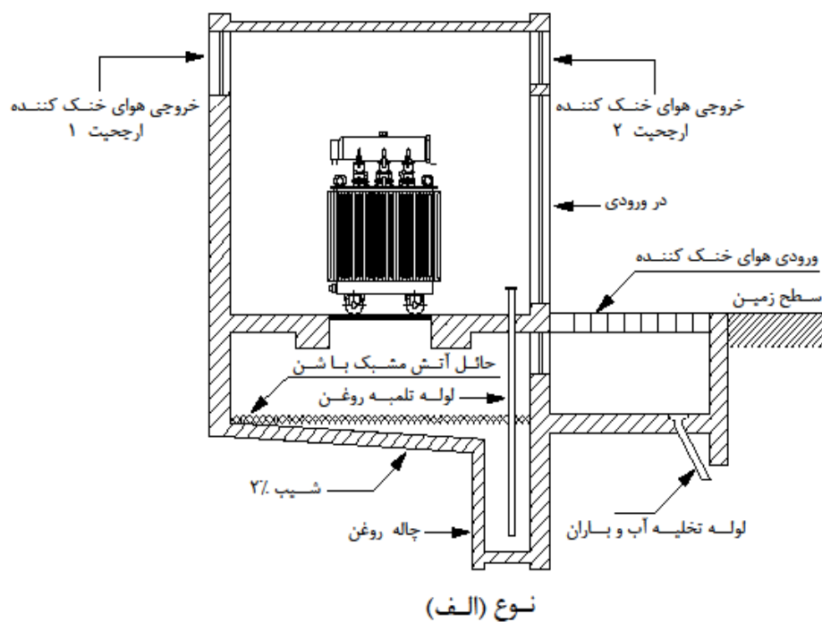
شکل ۵-۱۳-۳-۲: نوع الف) - طرحواره مقطع قائم اتاق ترانسفورماتور روغنی با تهویه مکانیکی و هم سطح زمین
