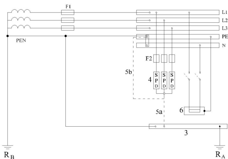
شکل ۱۳-۳-۱-۱۶-۱:۴ طرحواره نصب برقگیر حفاظتی در شبکه توزیع سیستم نیروی TN (سه فاز)
