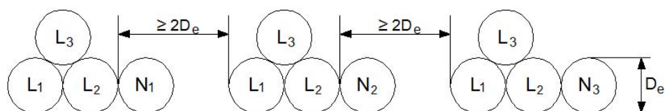
شکل ۷-۱۳-۱-۷-۱: آرایش مثلثی مخصوص برای رشته کابل تک رشته موازی (سه فاز)
