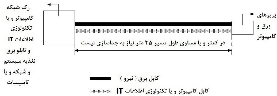
شکل ۱۳-۳-۱: ۱: طرحواره مسیر مشترک کابل برق و کابل کامپیوتر یا فناوری اطلاعات IT برای طول مسیر کمتر یا مساوی ۳۵ متر
