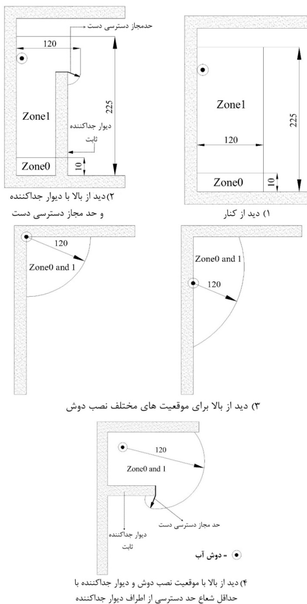
شکل ۱۳-۱۰-۴-۲: طرحواره موقعیت و ابعاد مناطق (zone) ها در حمام بدون زیردوشی
