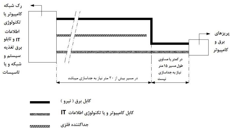
شکل ۱۳-۳-۲: ۲: طرحواره مسیر مجزا و مشترک کابل برق و کابل کامپیوتر یا فناوری اطلاعات IT برای طول مسیر بیش از ۳۵ متر
