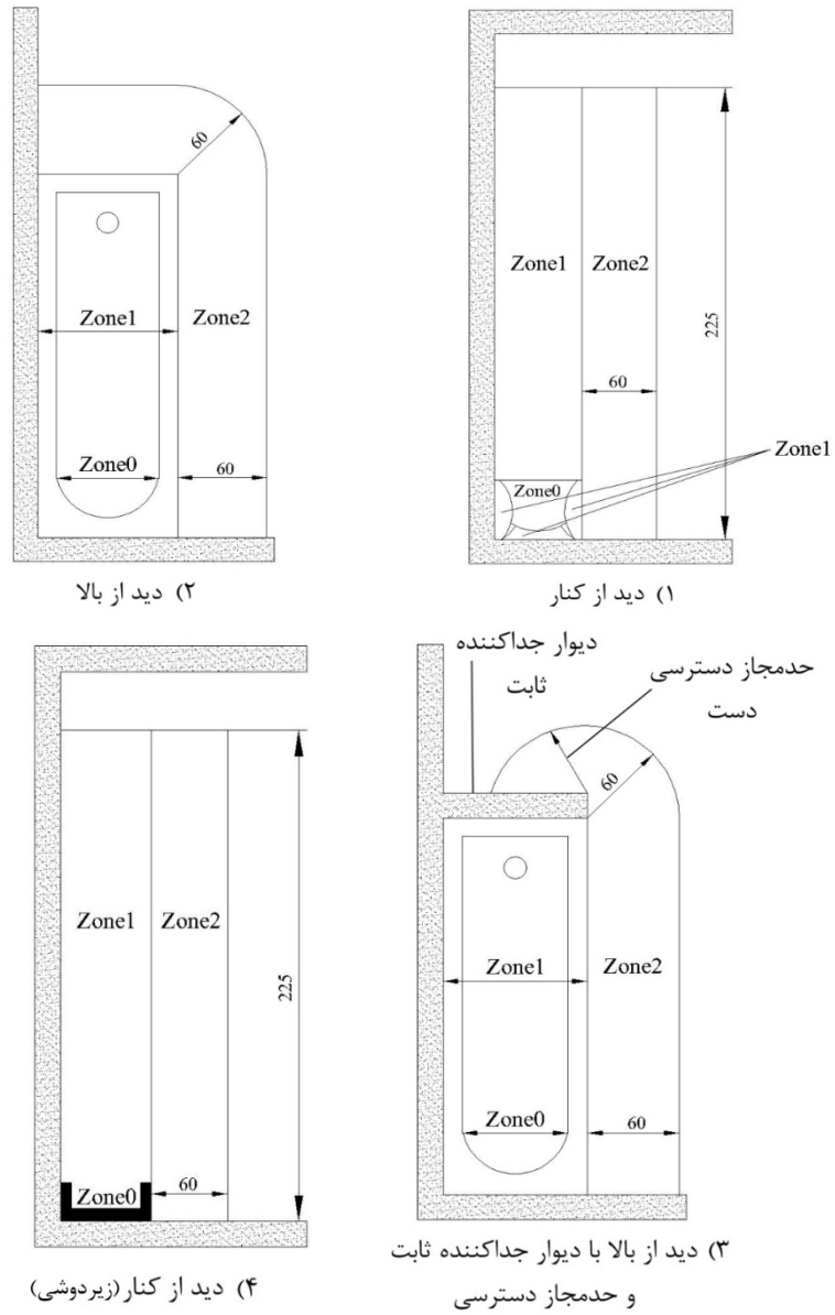
شکل ۱۰-۴-۱۳: طرحواره موقعیت و ابعاد مناطق (zone) ها یا موقعیت زیردوش
