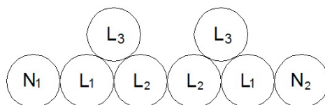
شکل ۱۳-۷-۳: آرایش مثلثی چسبیده به هم برای ۶ رشته کابل تک‌رشته موازی (سه‌فاز)
