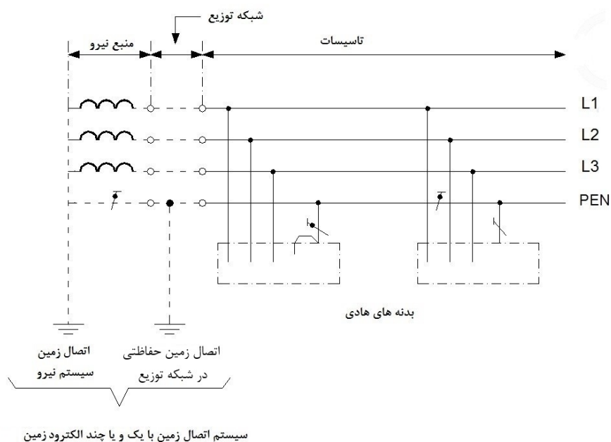
شکل پ ۱-۱:۲ سیستم TN-C در سیستم سه فاز چهار سیمه با هادی مشترک حفاظتی - خنثی در سرتاسر سیستم
