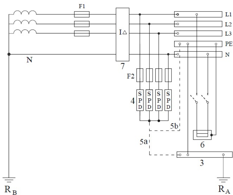
شکل ۱۳-۳-۱-۱۶-۲:۴ طرحواره نصب برقگیر حفاظتی در شبکه توزیع سیستم نیروی TT با قرارگیری برقگیر حفاظتی در طرف تغذیه بار و بعد از کلید حفاظتی جریان باقی مانده (RCD)
