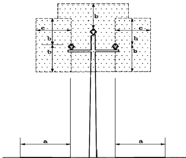
شکل پ ۱:۱-۲-۷ خط هوایی فشار متوسط (۱۱، ۲۰ و ۳۳ کیلوولت)
