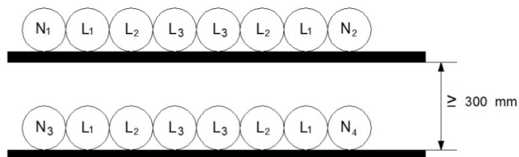
شکل ۷-۱۳-۱-۷-۱: آرایش چسبیده به هم در دو تراز به فاصله ۳۰ سانتی متر از هم برای ۱۲ رشته کابل تک رشته موازی (سه فاز)
