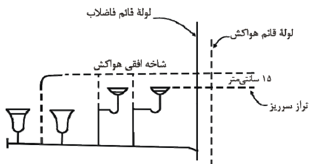
شکل ۵-۱۶-۲-۵ "پ" (۲) - اتصال هواکش به شاخه افقی لوله فاضلاب
